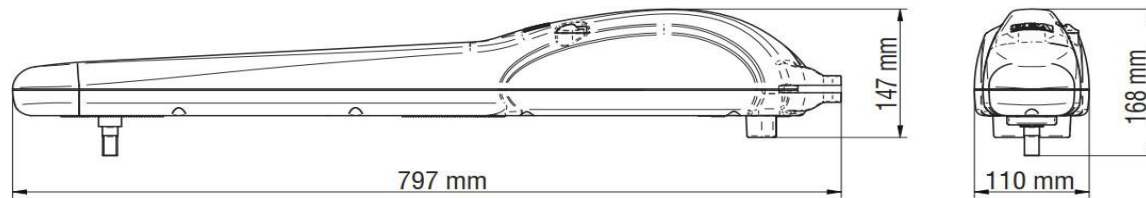
Kích thước motor tay đòn STING
