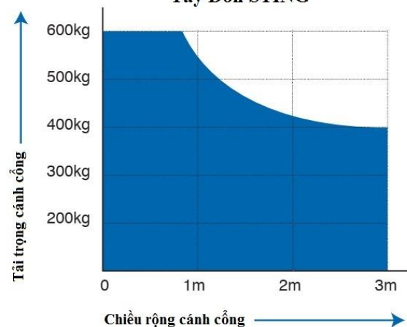
Biểu Đồ Lực Tay Đòn STING
